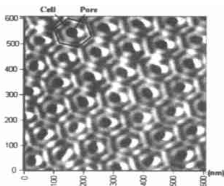
图1 多孔氧化铝模板(Porous Alumina Membranes)的AFM图像
