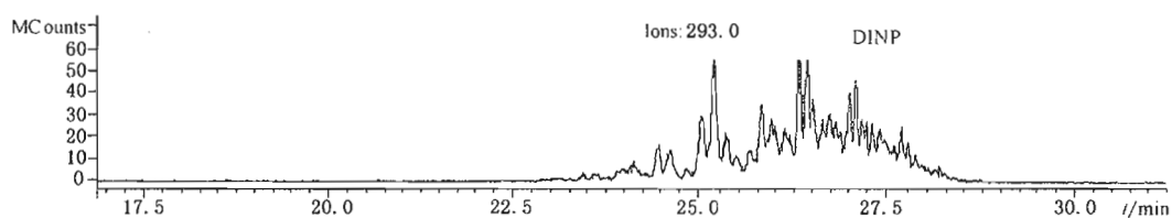
图 C.2 邻苯二甲酸二异壬酯 diisononylphthalate (DINP)(25.7~28.6 min)的提取离子色谱图
