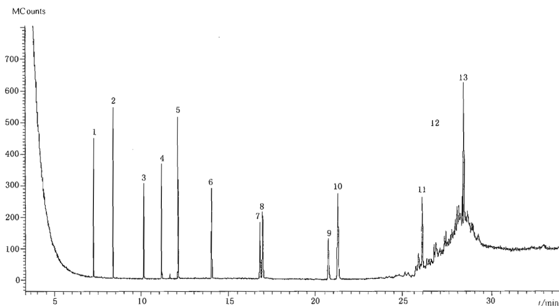
12 种邻苯二甲酸酯类增塑剂标准品的总离子流色谱图
