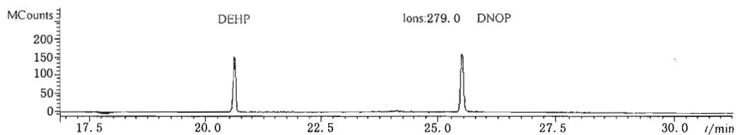
图 C.1 邻苯二甲酸二正辛酯 di-n-octylphthalate (DNOP)(26.1 min)的提取离子色谱图
