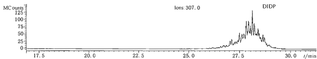
图 C.3 邻苯二甲酸二异癸酯 diisodecylphthalate (DIDP)(27.1~29.2 min)的提取离子色谱图
